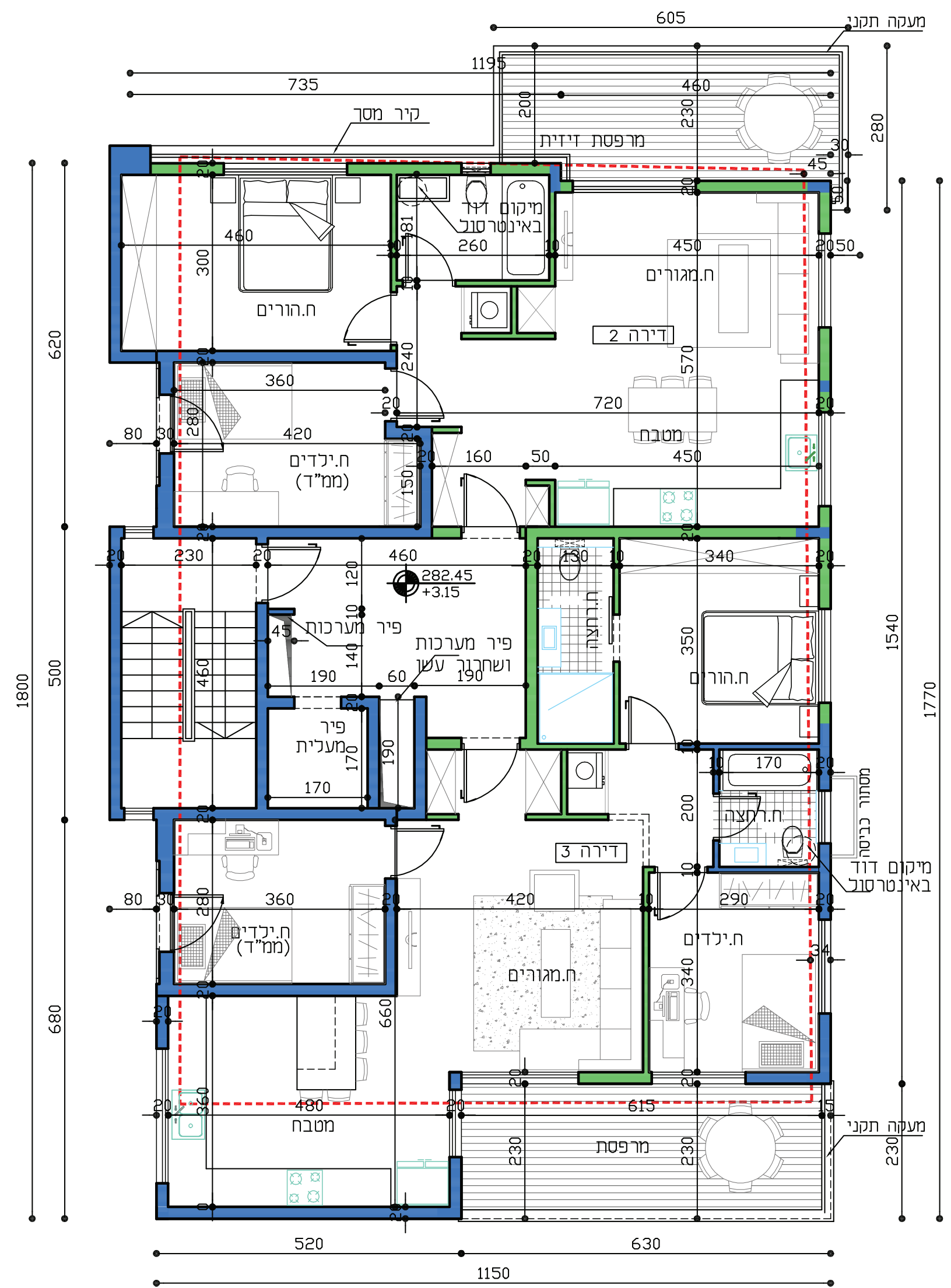
תוכנית קומה אי קני"מ 1:100
