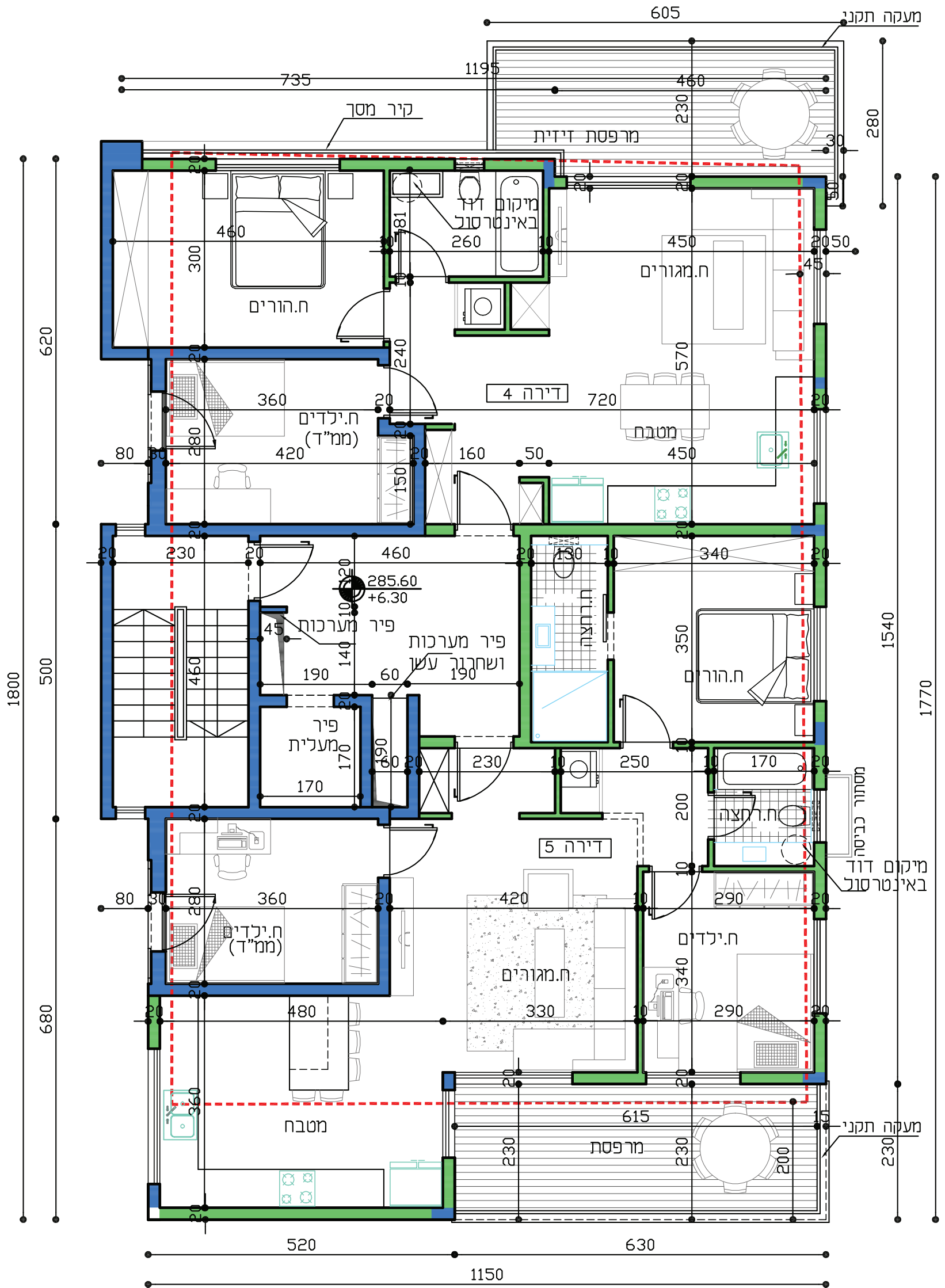
תוכנית קומה ב' קנ"מ 1:100
